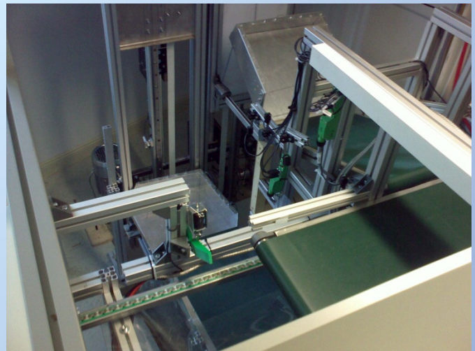
Hihnakuljetin ja siirtohissit
