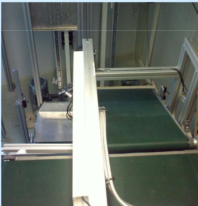
Hihnakuuljetin ja siirtohisit
