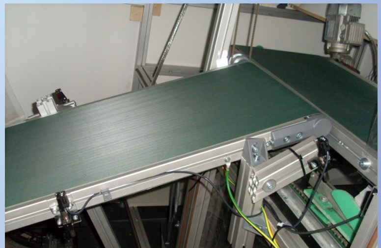
Hihnakuuljetin siirtohisiltä
